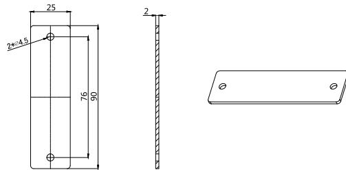
2.0406.0001 Fixation pour moteur AM55
