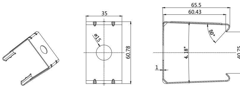
2.0406.0004 Fixation pour moteur AM55
