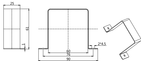
2.0406.0002 Fixation pour moteur AM55
