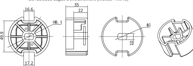
1.0405.0065 Bague d'entraînement (Moteur AM45)
