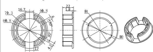
1.0405.0026 Bague de fin de course(Moteur AM45)
