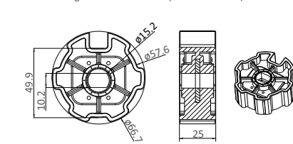
1.0405.0097 Bague d'entraînement (Moteur AM45)
