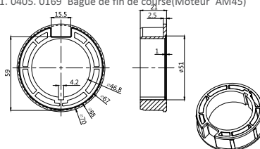
1.0405.0170 Bague d'entraînement (Moteur AM45)
