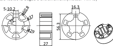
1.0405.0045 Bague d'entraînement (Moteur AM45)
