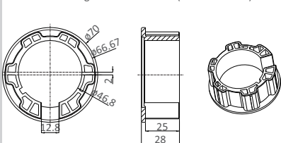
1.0405.0096 Bague de fin de course(Moteur AM45)
