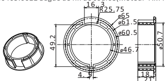
1.0405.0022 Bague de fin de course(Moteur AM45)
