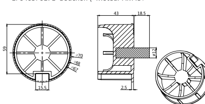
1.0405.0171 Bouchon ( Moteur AM45)
