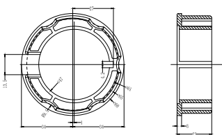
1.0405.0009 Bague de fin de course(Moteur AM45)
