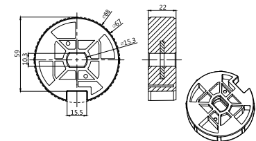
1.0405.0171 Bouchon ( Moteur AM45)
