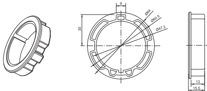
1.0405.0010 Bague de fin de course(Moteur AM45)
