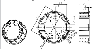
1.0405.0096 Bague de fin de course(Moteur AM45)
