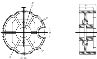
1.0405.0043 Bague d'entraînement (Moteur AM45)
