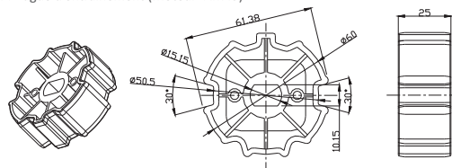
1.0405.0044 Bague d'entraînement (Moteur AM45)
