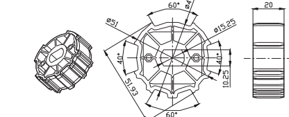
1.0404.0052 Bague d'entraînement (Moteur AM35)
