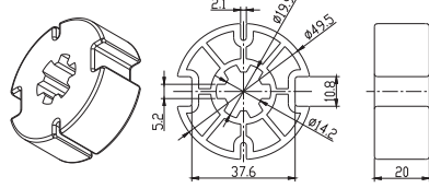
1.0404.0048 Bague d'entraînement (Moteur AM35)
