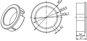
1.0404.0015 Bague de fin de course (Moteur AM35)
