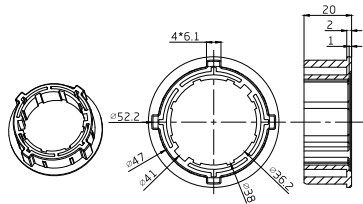
1.0404.0152 Bague de fin de course (Moteur AM35)
