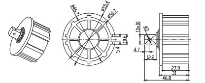
7.1000.0071 Bouchon (sans roulement)
