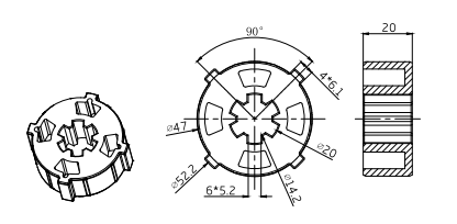
1.0404.0154 Bague d'entraînement (Moteur AM35)
