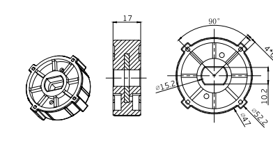
1.0404.0153 Bague d'entraînement (Moteur AM35)
