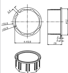
1.0405.0136 Bague de fin de course (Moteur AM45)
