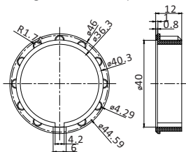
1.0404.0008 Bague de fin de course (Moteur AM35)
