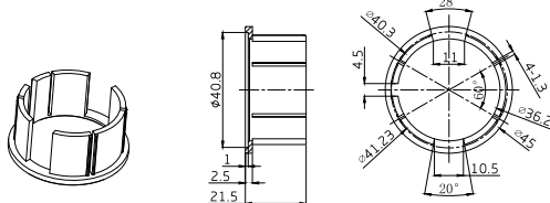
1.0404.0131 Bague de fin de course (Moteur AM35)
