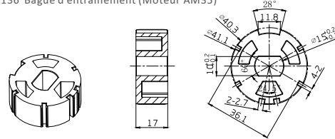
1.0404.0132 Bague d'entraînement (Moteur AM35)
