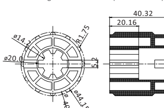
1.0404.0041 Bague d'entraînement (Moteur AM35)
