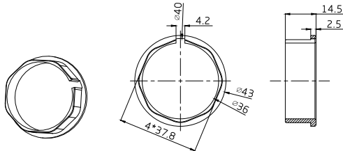
1.0404.0131 Bague de fin de course (Moteur AM35)
