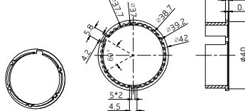
1.0404.0162 Bague de fin de course (Moteur AM35)
