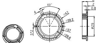
1.0404.0162 Bague de fin de course (Moteur AM35)
