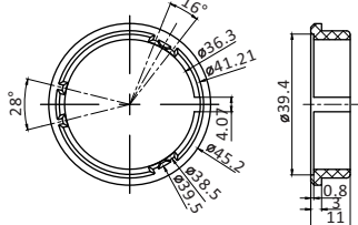
1.0404.0007 Bague de fin de course (Moteur AM35)
