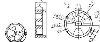
1.0404.0163 Bague d'entraînement (Moteur AM35)
