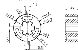
1.0404.0163 Bague d'entraînement (Moteur AM35)
