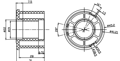
1.0403.0053 Bouchon (Moteur AM35)
