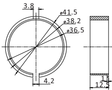
1.0404.0141 Bague de fin de course (Moteur AM35)
