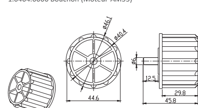
1.0404.0066 Bouchon (Moteur AM35)
