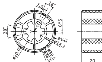
1.0404.0040 Bague d'entraînement (Moteur AM35)
